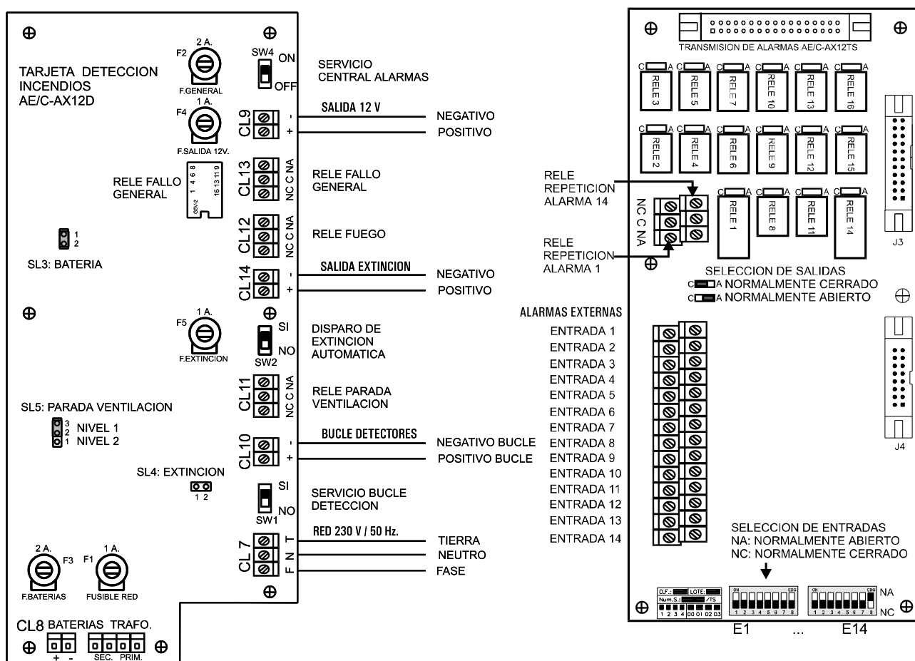
Fig.: 1 Esquema general de conexión.
