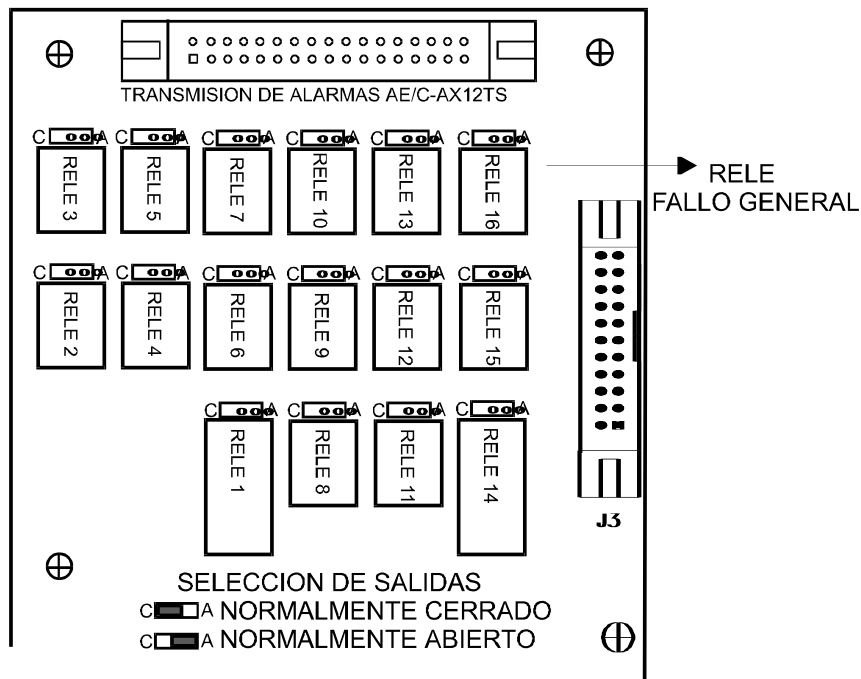
Fig.: 7 Tarjeta de transmisión de alarmas.
