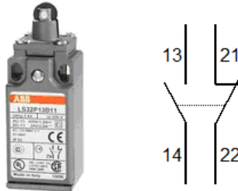
Figura 14: Final de carrera.
