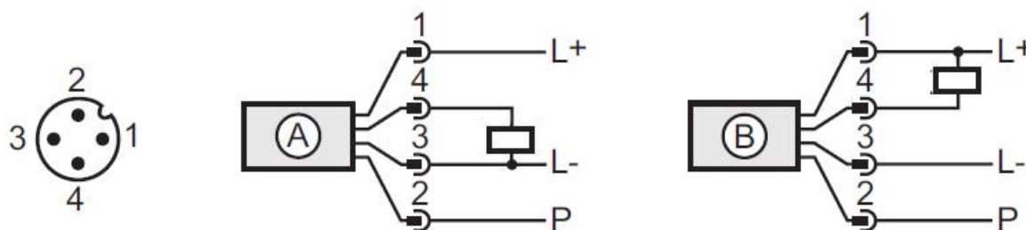
Figura 2: Conexión eléctrica.
