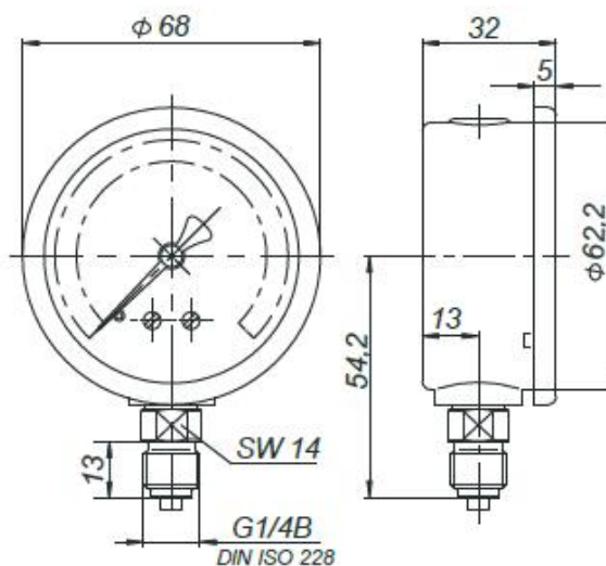
Figura 14: Dimensiones manómetro tecsis serie1454.
